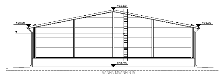
JULKISIVU ETELÄÄN
