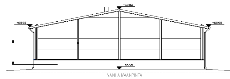
JULKISIVU POHJOISEEN
