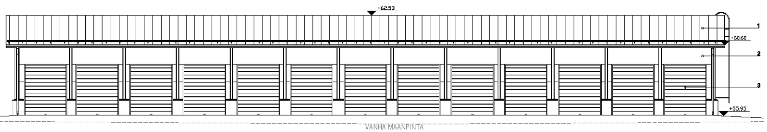
JULKISIVU LÄNTEEN
